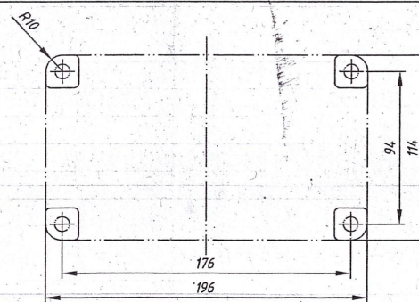
图2 减速器安装平台示意图
